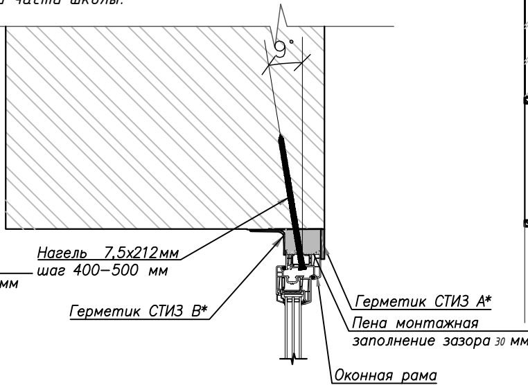
Крепление оконной рамы к перемычкам оконных проемов новой части школы.
