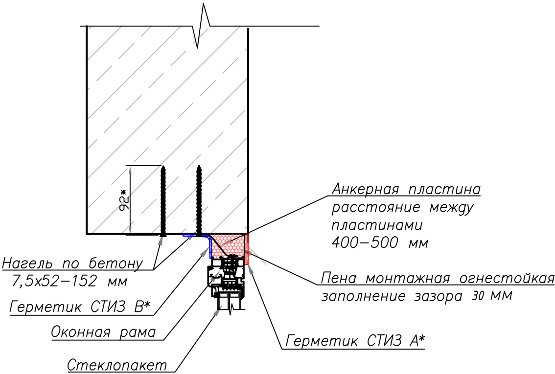
Узел примыкания к потолочному откосу проема рамы огнестойкого оконного блока
