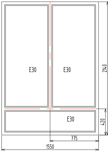
ОК-4/1 E30 (3-4-эт)
