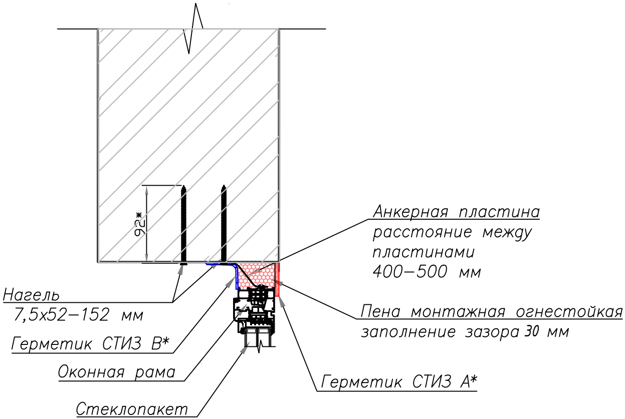
Узел примыкания к потолочному откоосу проема рамы огнестойкого оконного блока
