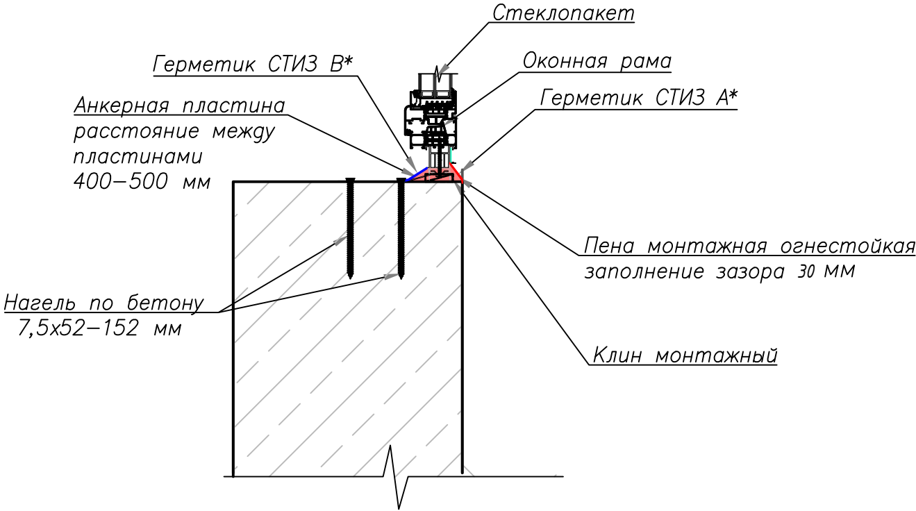
Узел примыкания к нижней части проема рамы огнестойкого оконного блока
