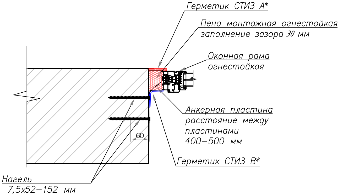
Узел примыкания к вертикальному участку проема рамы огнестойкого оконного блока (вид сверху)
