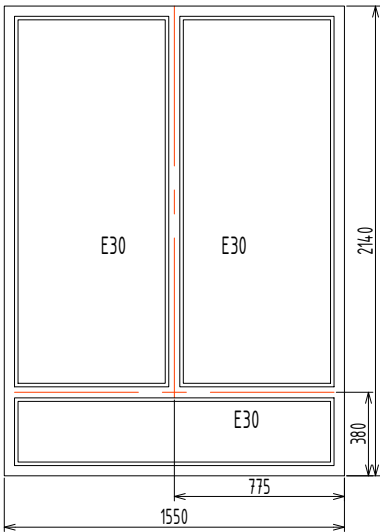
ОК-4/1 E30 (1-2-эт)
