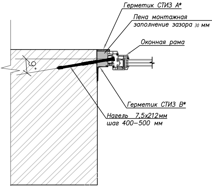
Крепление оконной рамы к вертикальным участкам проемов. Вариант 2 (вид сверху)
