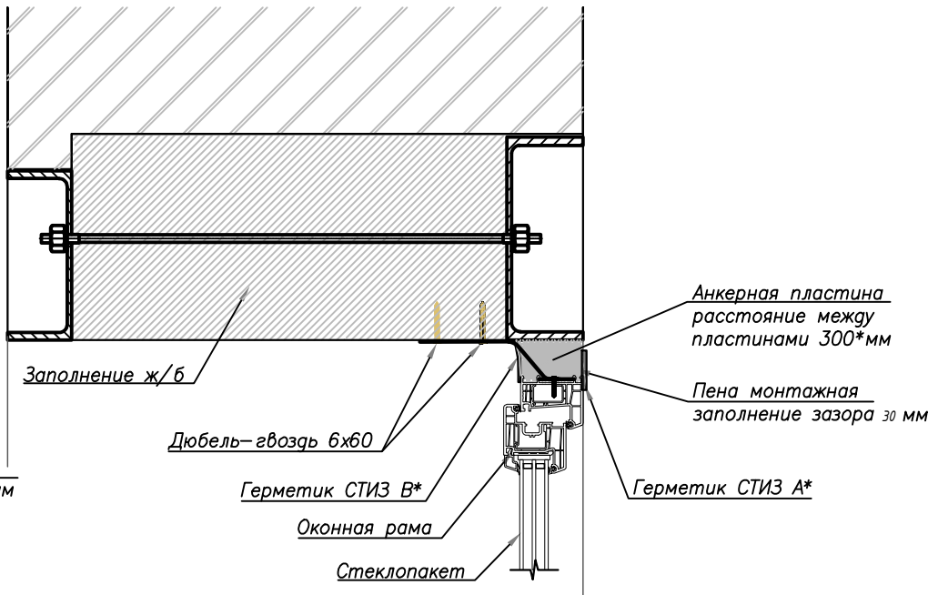
Крепление оконной рамы к перемычкам оконных проемов старой части школы. Вариант 2 (вид сбоку)
