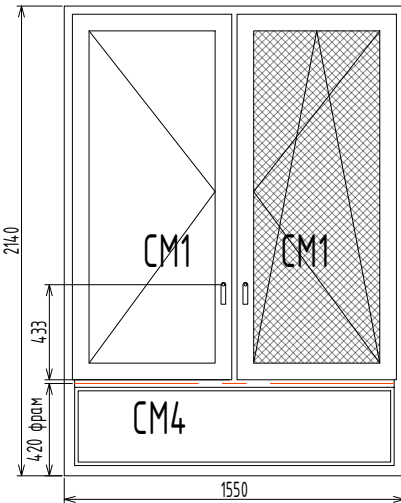
ОК-4/3 (3-4-эт) ОК-4 (3-4-эт)
