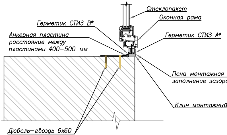
Крепление оконной рамы в нижней части проема
