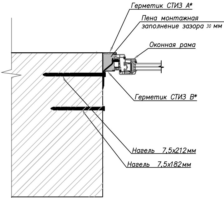
Крепление оконной рамы к вертикальным участкам проемов. Вариант 1 (вид сверху)
