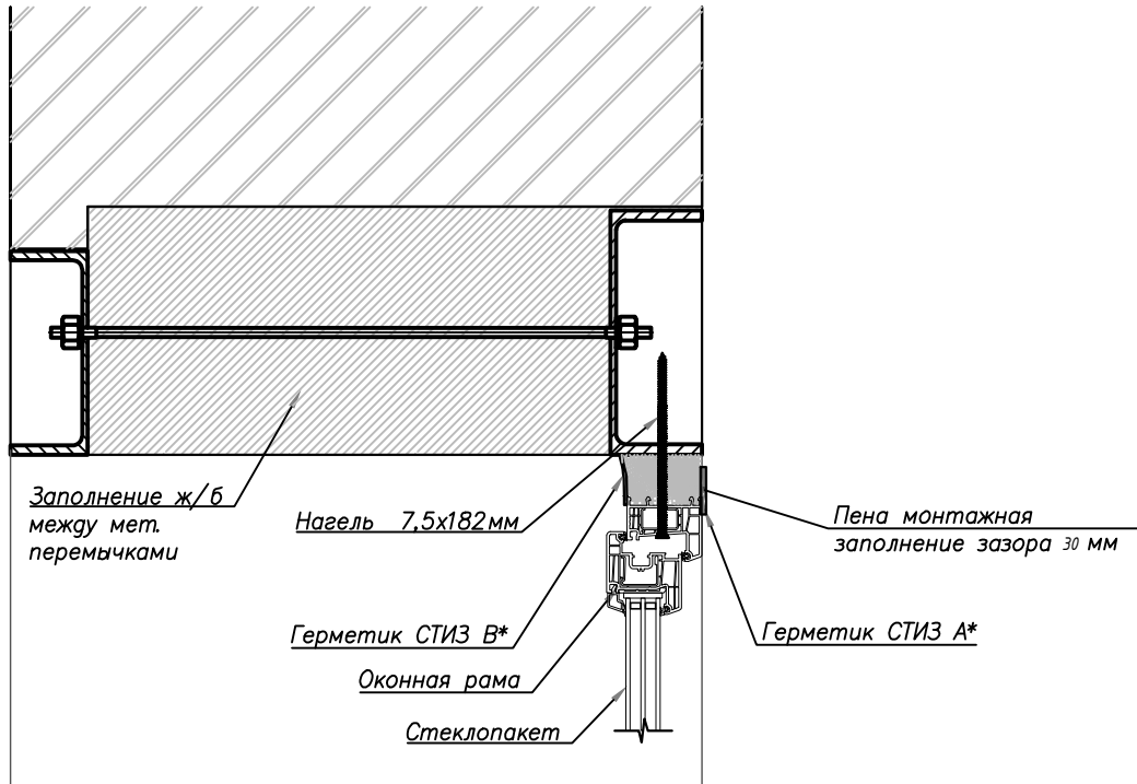
Крепление оконной рамы к перемычкам оконных проемов старой части школы. Вариант 2 (вид сбоку)
